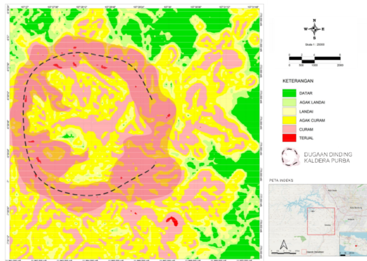
Gambar 4. Peta Kelerengan berdasarkan Klasifikasi ITC (Van Zuidam, 1977)
