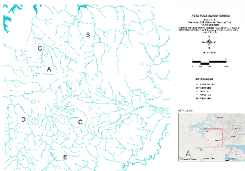
Gambar 3. Pola Pengaliran Sungai
