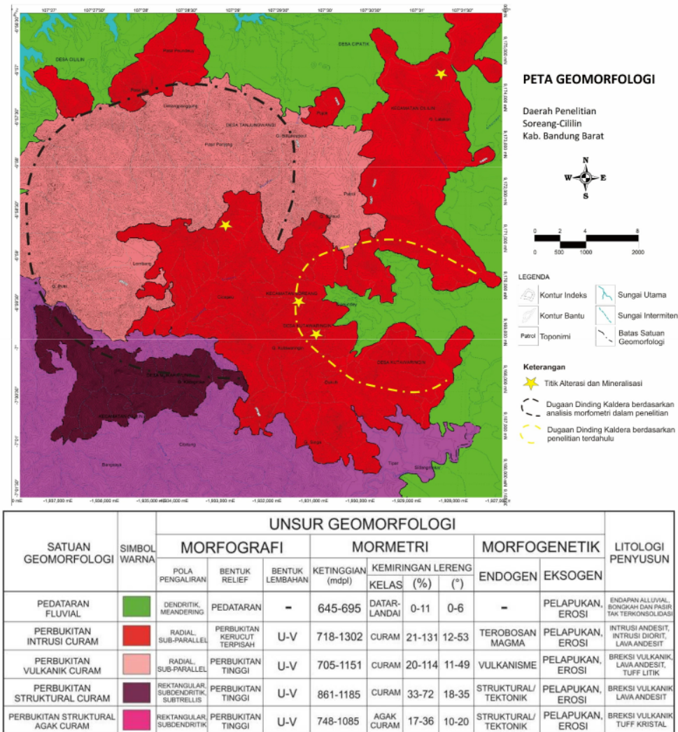
Gambar 5. Peta Geomorfologi Daerah Penelitian dan Pembagian Satuan Geomorfologi Berdasarkan Aspek Morfografi, Mormetri, dan Morfogenetik.
