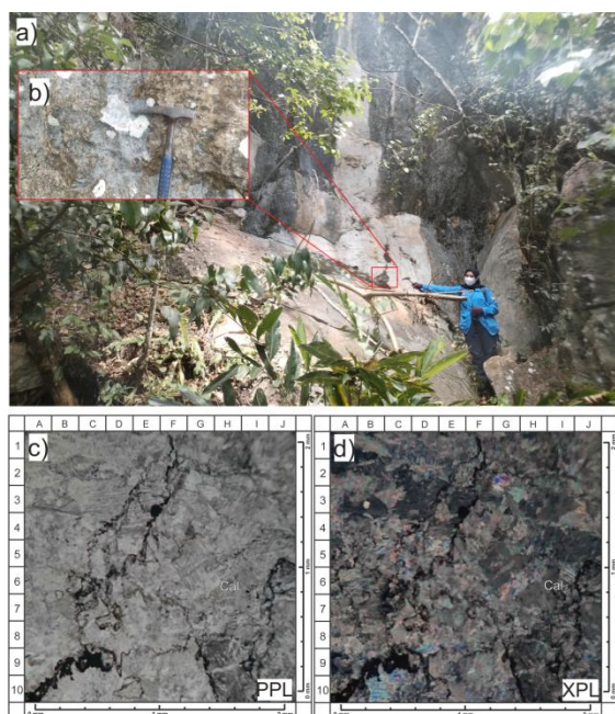
Gambar 6. a) Singkapan Batugamping Kristalin, b) Batugamping Kristalin, c) Sayatan Nikol Sejajar, d) Sayatan Nikol Silang.
