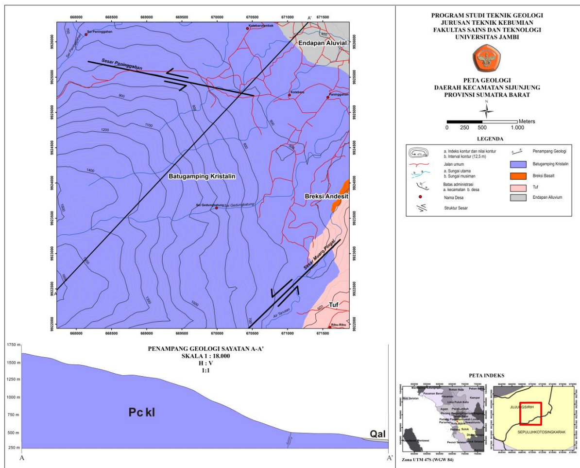
Gambar 4. Peta Geologi.
