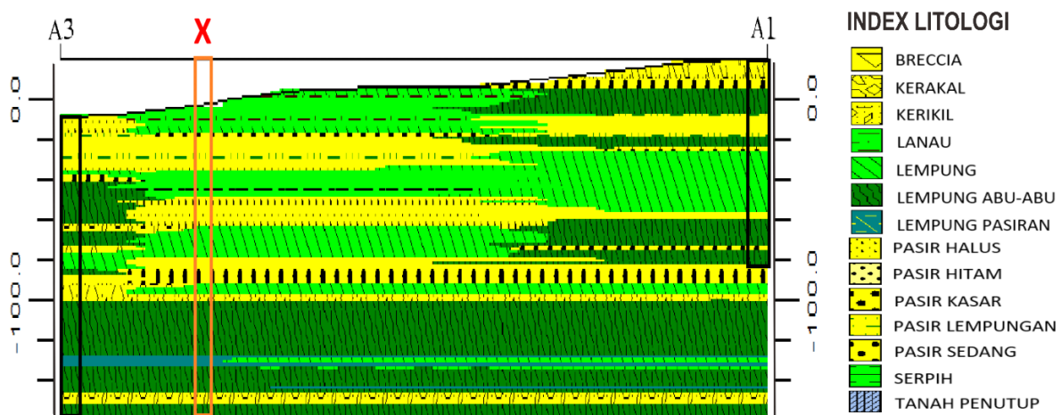
Gambar 5. Cross Section Litologi pada Lintasan B teatnya di sumur A3-A1.
