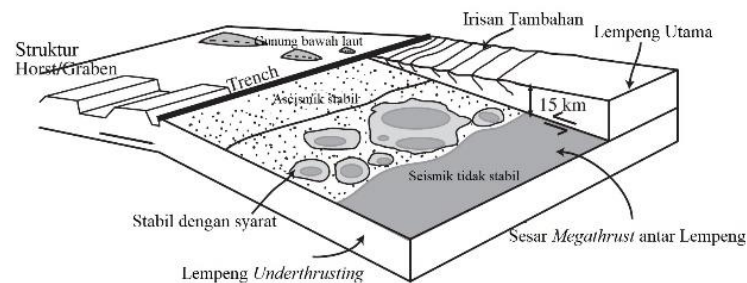
Gambar 4. Model Lempeng pada Zona Subduksi pemacu gempabumi dangkal di bawah laut (Bilek & Lay, 2002).
