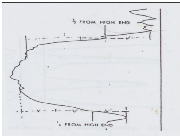
Gambar 3. Penentuan ketebalan menggunakan log gamma ray (BPB Manual, 1981).
