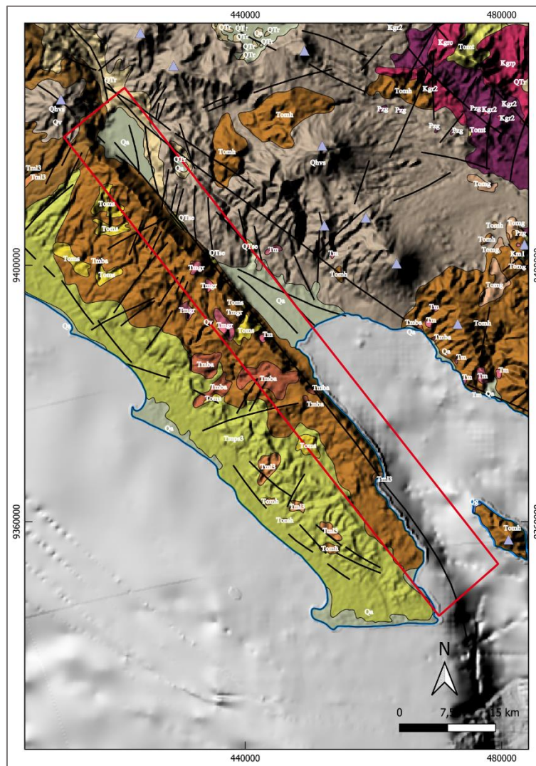
Gambar 3. Peta geologi di area penelitian (Amin dkk., 1993). Area penelitian ditandai persegi Panjang berwarna merah.
