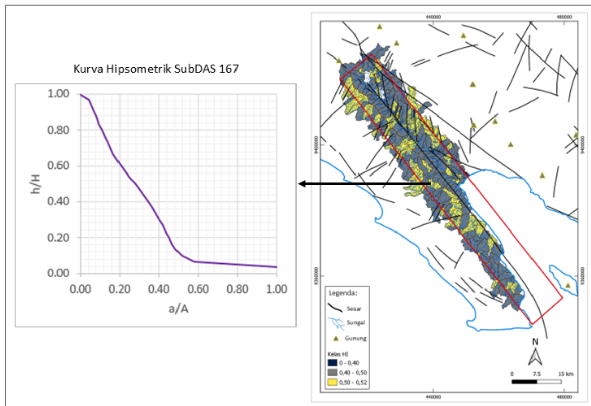
Gambar 9. Anomali kurva hipsometrik SubDAS 167 di Zona Sesar Semangko.
