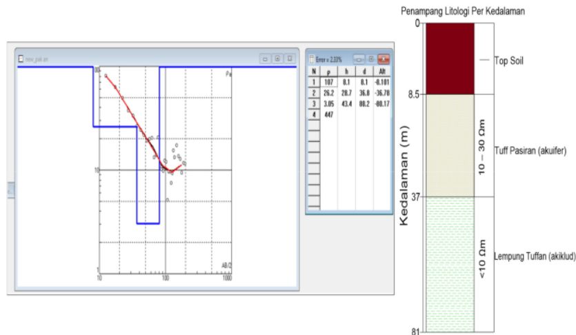
Gambar 9. Hasil pengukuran dari VES PKM_S5 memperlihatkan model resistivitas pada gambar sebelah kiri dan hasil interpretasi pada gambar sebelah kanan.
