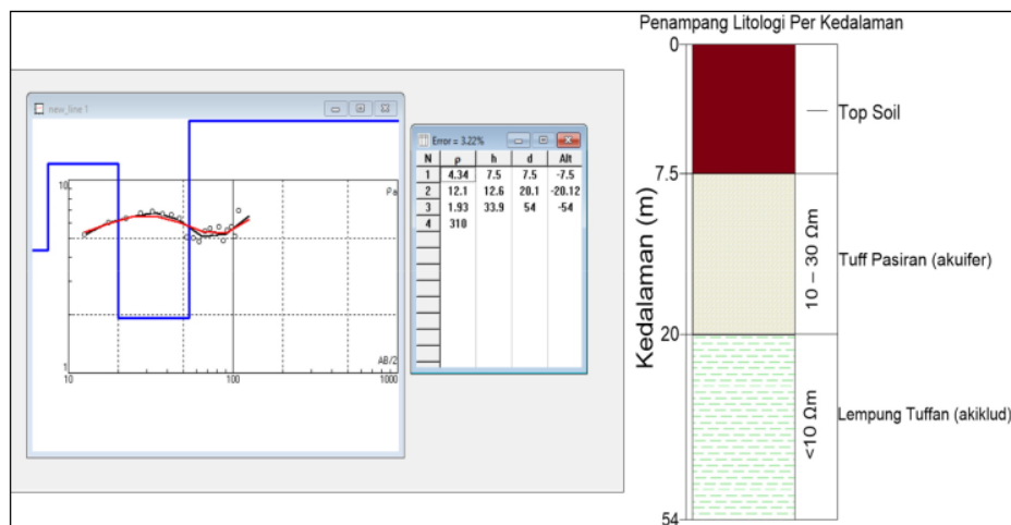
Gambar 4. Hasil pengukuran dari titik PKM_S1 memperlihatkan model resistivitas pada gambar sebelah kiri dan hasil interpretasi pada gambar sebelah kanan.
