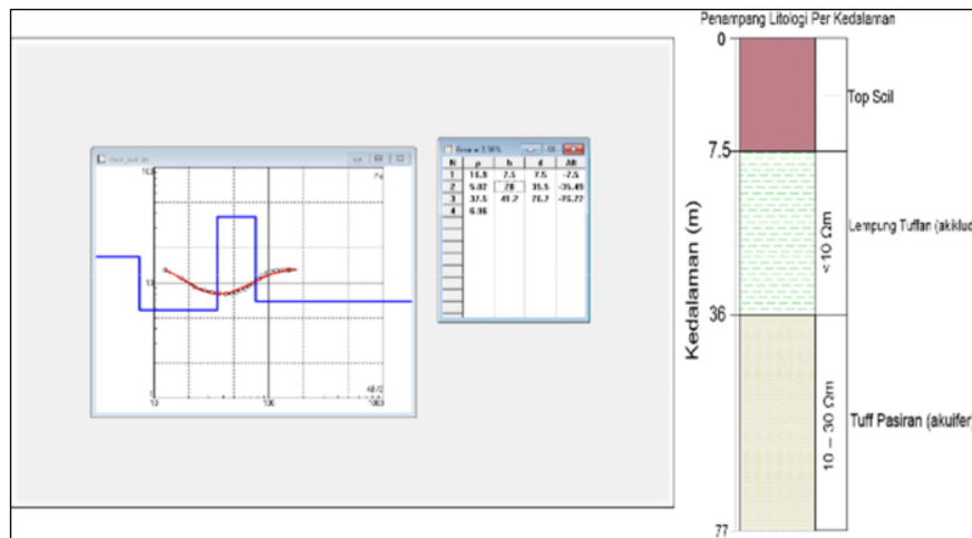
Gambar 8 Hasil pengukuran dari VES PKM_S4 memperlihatkan model resistivitas pada gambar sebelah kiri dan hasil interpretasi pada gambar sebelah kanan.
