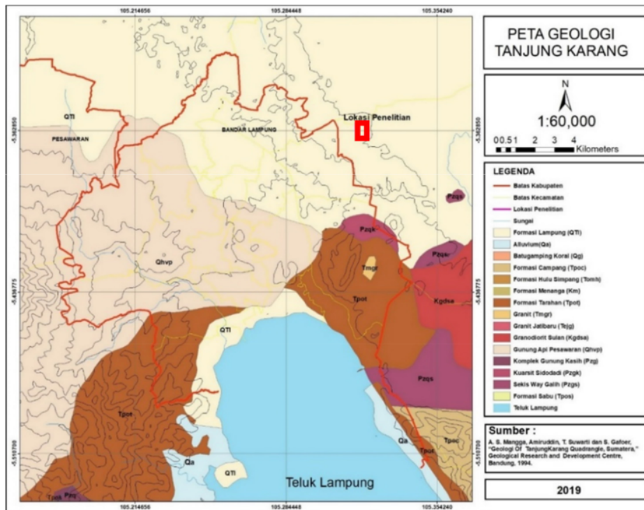
Gambar 3 Peta geologi daerah penelitian (modifikasi dari Mangga dkk., 1993).
