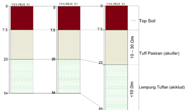
Gambar 7. Korelasi tiga titik pengukuran PKM_S1, PKM_S2 dan PKM_S3.
