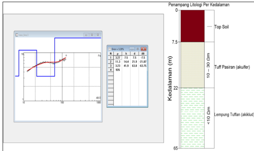
Gambar 6. Hasil pengukuran dari titik VES PKM_S3 memperlihatkan model resistivitas pada gambar sebelah kiri dan hasil interpretasi pada gambar sebelah kanan.
