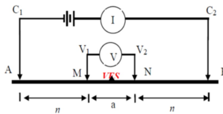
Gambar 2. Susunan Elektroda Konfigurasi Schlumberger (Dimodifikasi dari Loke, 2016).
