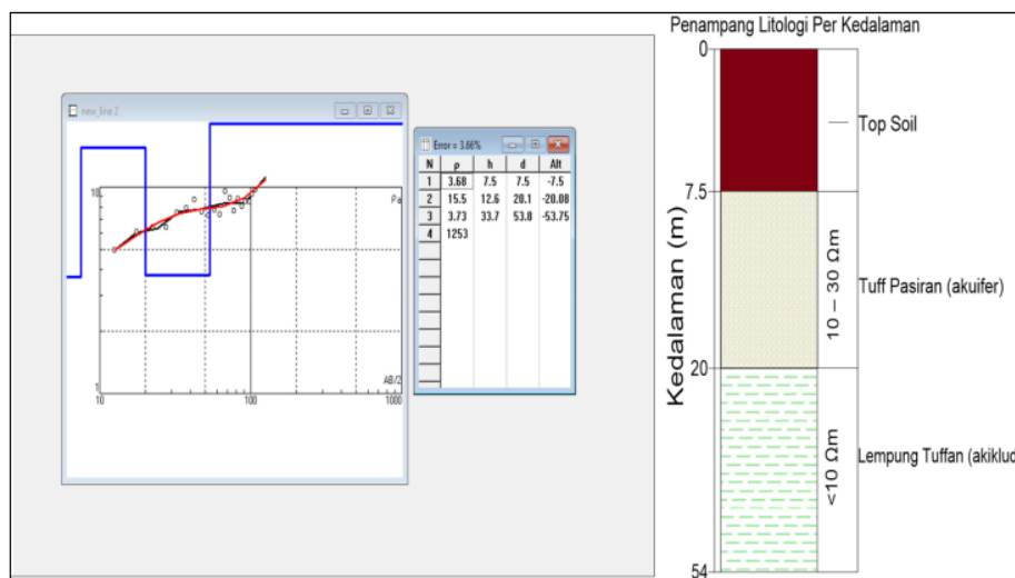
Gambar 5. Hasil pengukuran dari titik VES PKM_S2 memperlihatkan model resistivitas pada gambar sebelah kiri dan hasil interpretasi pada gambar sebelah kanan.
