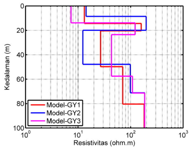
Gambar 5. Profil resistivitas terhadap kedalaman hasil inversi.
