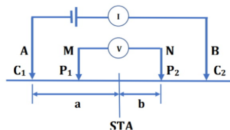
Gambar 3. Layout pengukuran metode geolistrik dengan teknik VES konfigurasi Schlumberger (Riska & Satiawan, 2019)
