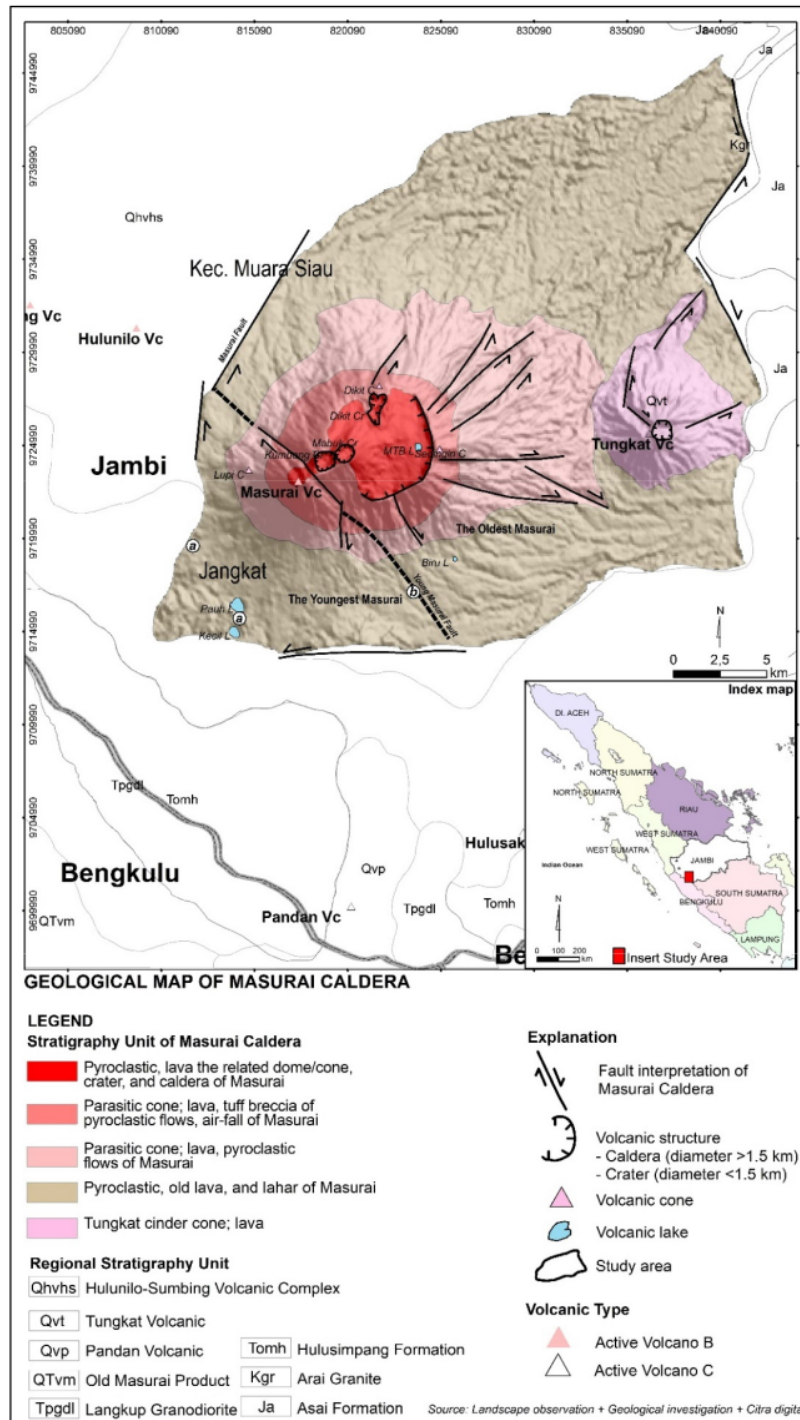
Gambar 7. Peta Geologi Kaldere Masurai
