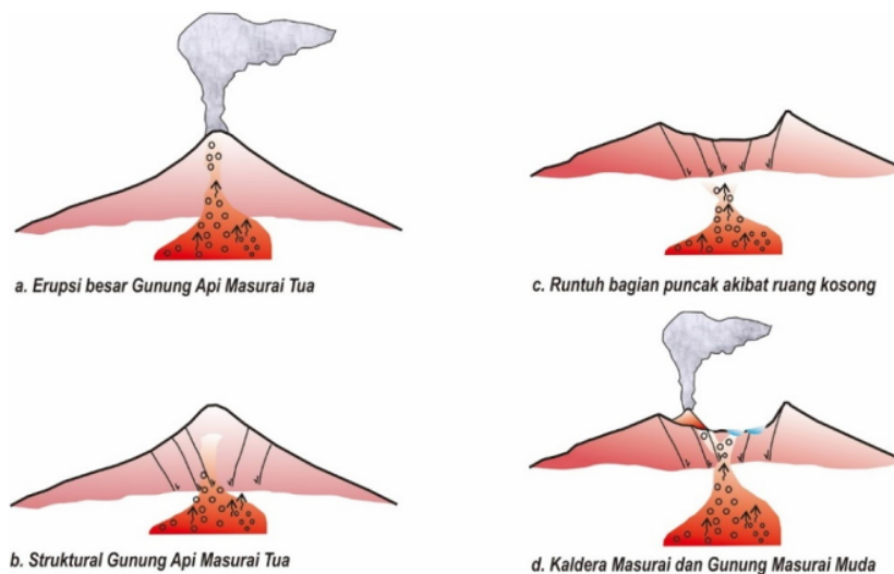
Gambar 6. Proses pembentukan Kaldera Masurai. (a) Erupsi besar Gunung Api Masurai Tua pada Plistosen Akhir, (b) Terjadinya mekanisme struktural pada morfologi puncak
