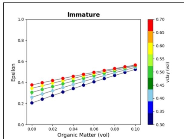
Gambar 3. Grafik parameter epsilon terhadap organic matter dengan variasi mineral.
