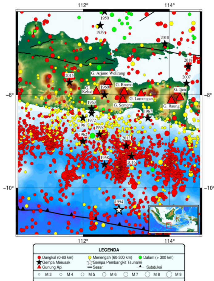
Gambar 1. Peta seismisitas Jawa Timur (BMKG, 2021).
