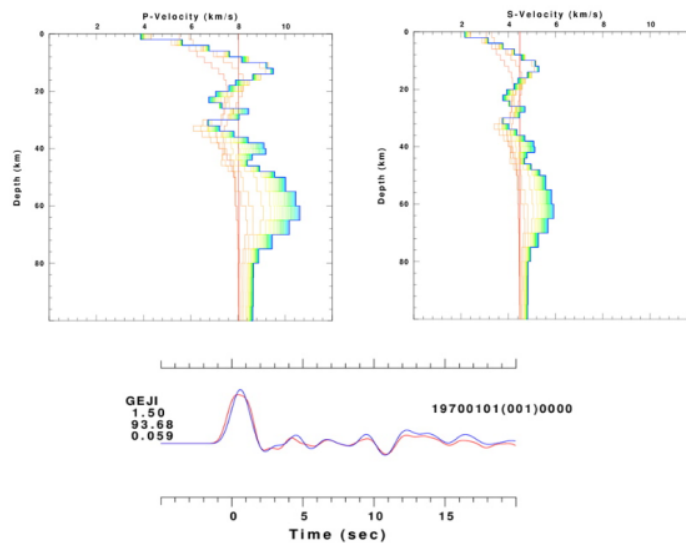
Gambar 19. Model kecepatan gelombang P (kiri) dan gelombang S (kanan) di bawah stasiun GEJI. Garis biru merupakan hasil akhir model kecepatan, garis merah merupakan model kecepatan awal, dan garis warna-warni merupakan proses iterasi model kecepatan. Panel bagian bawah merupakan fitting fungsi penerima observasi dan model digambarkan oleh garis biru dan merah.
