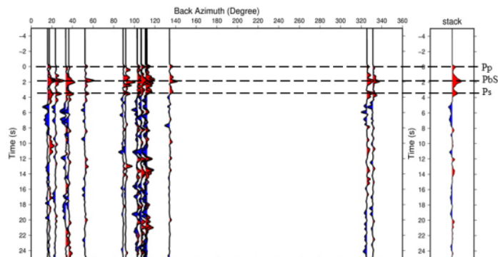
Gambar 6. Hasil sinyal fungsi penerima pada stasiun TBJI dengan nilai lebar filter Gaussian 5 ( \alpha = 5 ).
