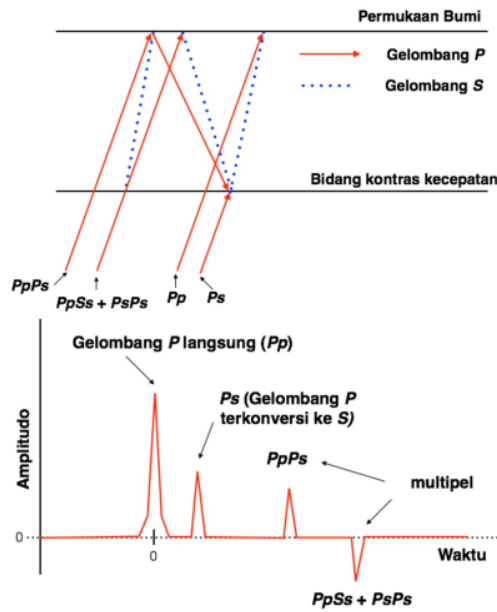
Gambar 2. Diagram fungsi penerima. Fasa konversi Ps dan fasa-fasa pantulannya (PpPs dan PpSs+PsPs) yang diterjemahkan dari bentuk suatu model lapisan bumi sederhana. Gambar dimodifikasi dari Ligorria (2000).
