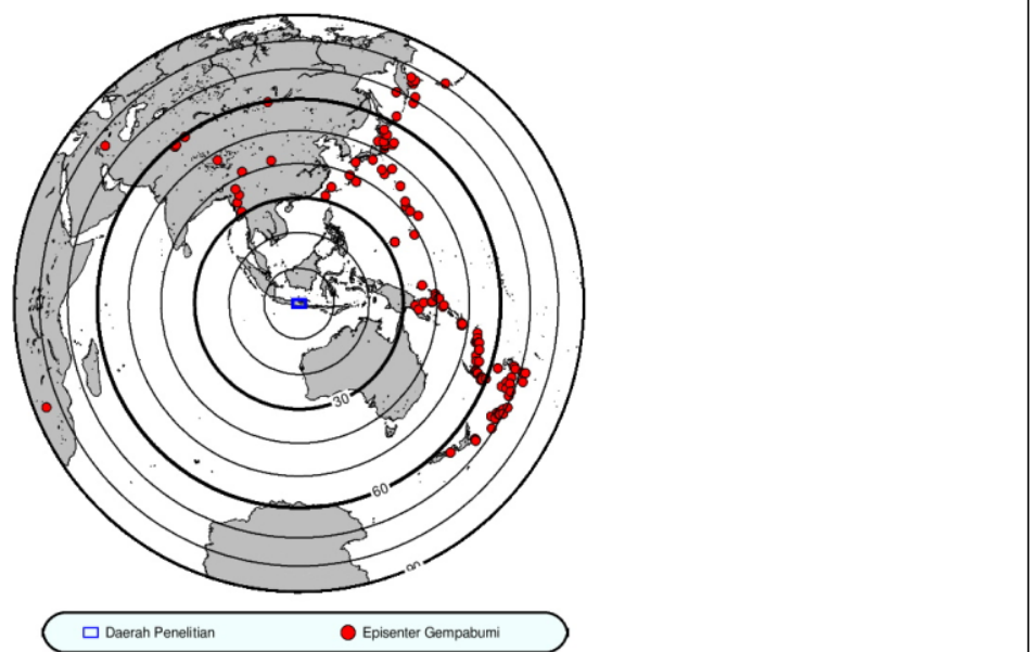
Gambar 4. Peta sebaran episenter gempabumi teleseismik yang digunakan.
