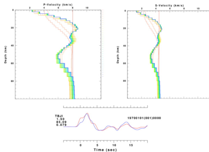
Gambar 7. Model kecepatan gelombang P (panel kiri atas) dan gelombang S (panel kanan atas) di bawah stasiun TBJI. Garis biru merupakan hasil akhir model kecepatan, garis merah merupakan model kecepatan awal, dan garis warna-warni merupakan proses iterasi model kecepatan. Panel bagian bawah merupakan fitting fungsi penerima observasi dan model digambarkan oleh garis biru dan merah.
