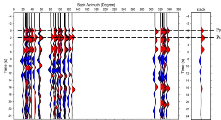
Gambar 12. Hasil fungsi penerima yang di plot berdasarkan back azimuth (kiri) dan hasil stacking (kanan) pada stasiun ABJI.
