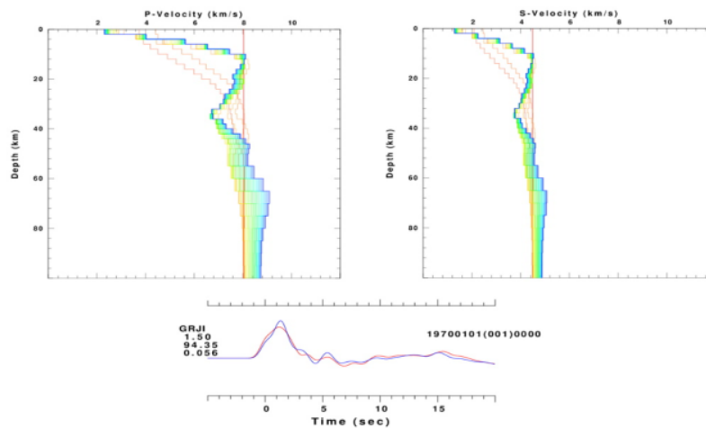
Gambar 8. Model kecepatan gelombang P (panel kiri atas) dan gelombang S (panel kanan atas) di bawah stasiun GRJI. Garis biru merupakan hasil akhir model kecepatan, garis merah merupakan model kecepatan awal, dan garis warna-warni merupakan proses iterasi model kecepatan. Panel bagian bawah merupakan fitting fungsi penerima observasi dan model digambarkan oleh garis biru dan merah.
