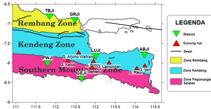
Gambar 3. Peta sebaran stasiun yang digunakan berdasarkan zona geologi utama di Jawa Timur (dimodifikasi dari Martha dkk. (2017)).
