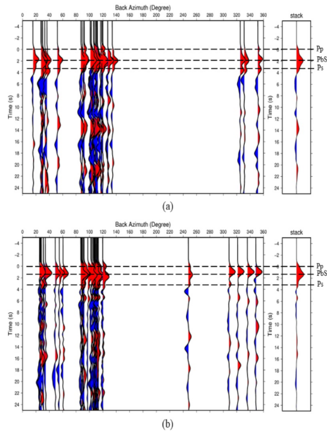
Gambar 5. Hasil fungsi penerima yang di plot berdasarkan back azimuth (kiri) dan hasil stacking (kanan) pada stasiun TBJI (a) dan stasiun GRJI (b)
