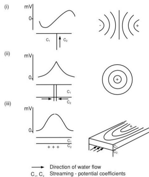
Gambar 1. Hubungan nilai anomaly self potential dengan arah aliran air: (i) batas vertikal sumur atas disebelah kanan; (ii) pompa dari sumur; (iii) batas horizontal aliran (Reynolds, 1997b).
