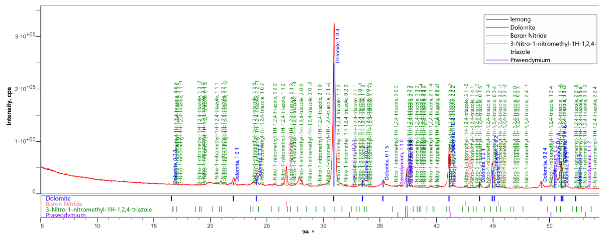
Gambar 1. Hasil Uji XRD Sampel Batuan Lemong
