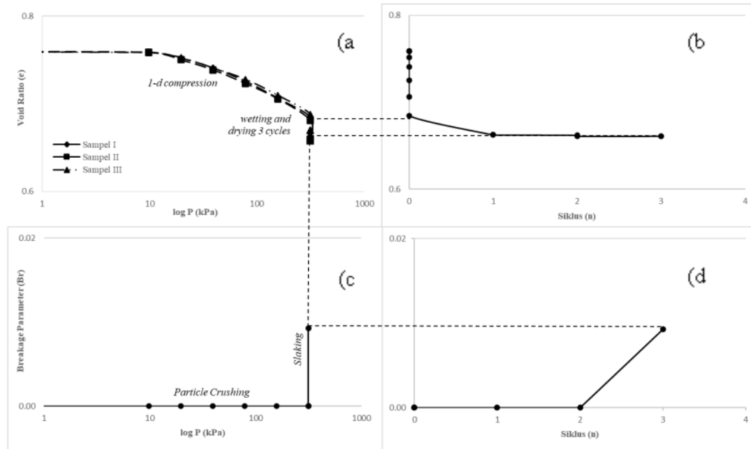
Gambar 6. Perubahan sifat tekan dan ukuran partikel batuan Lemong selama pengujian 1D Compression Slaking Test .
