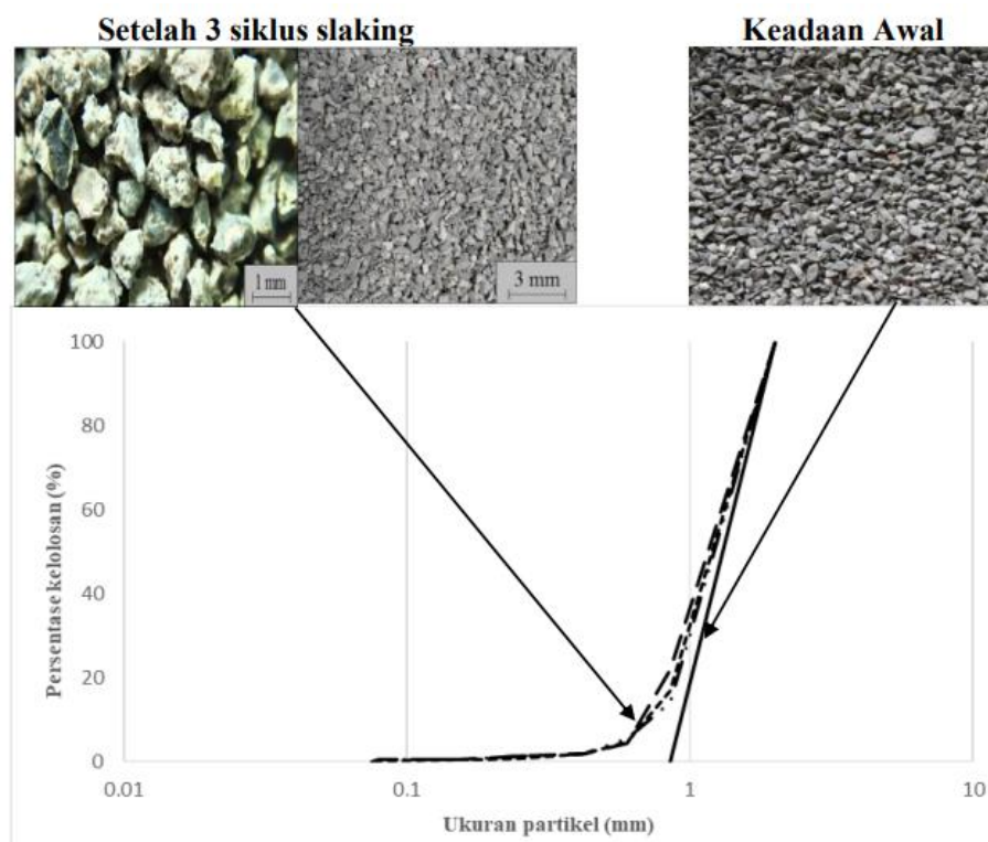
Gambar 5. Distribusi ukuran partikel batuan Lemong.
