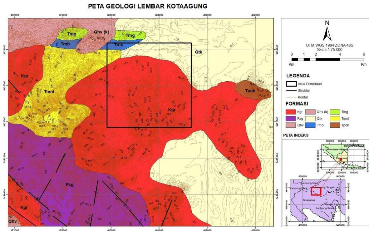
Gambar 2.1. Peta Geologi Lembar Kotaagung (Amin dkk., 1993) modifikasi.
