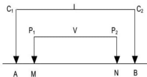
Gambar 4. Konfigurasi Schlumberger (Reynolds, 1998).
