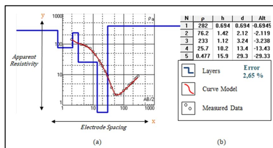
Gambar 7. Kurva dan tabel resistivitas per lapisan. Titik 2
