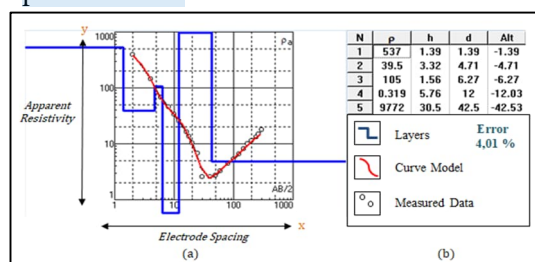
Gambar 6. Kurva dan tabel resistivitas titik 1.
