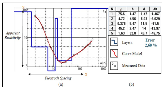
Gambar 10. Kurva tabel resistivitas Titik 5
